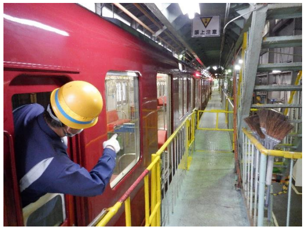
扉開閉試験
