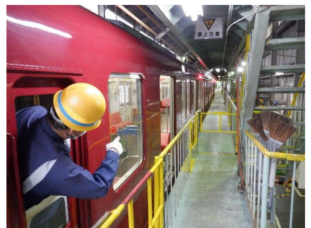
扉開閉試験
